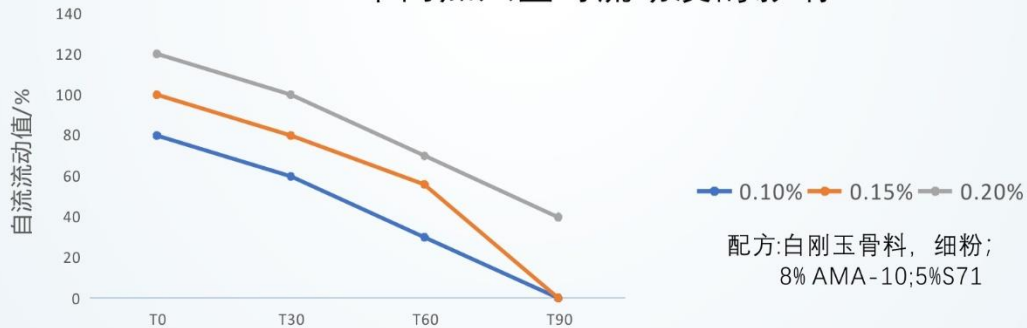
WSM-M不同加入量对流动度的影响
