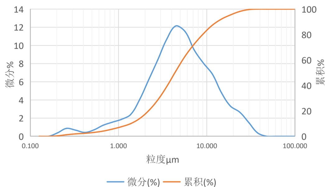
AMA-40 粒度分布曲线图
