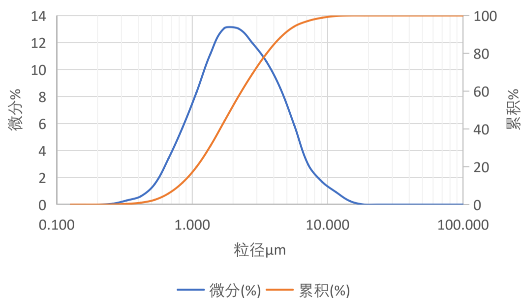
AMA-25 粒度分布曲线图
