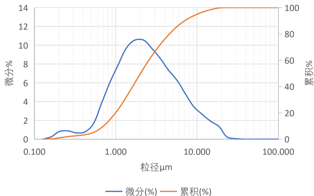
AMA-20粒度分布曲线图
