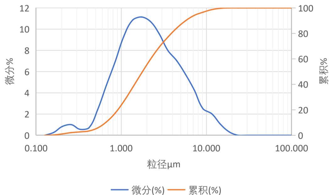
AMA-10 粒度分布曲线图
